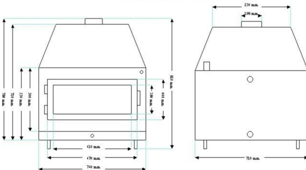
Wymiary poglądowe kominka 16 kW
