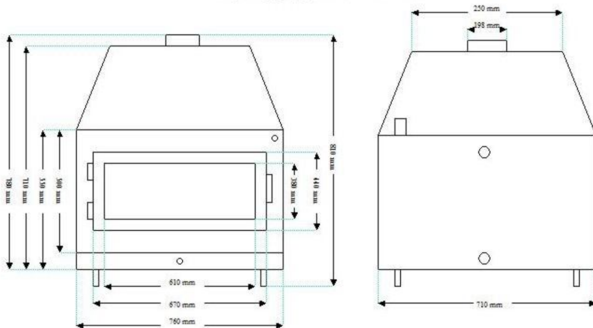
Wymiary poglądowe kominka 20 kW
