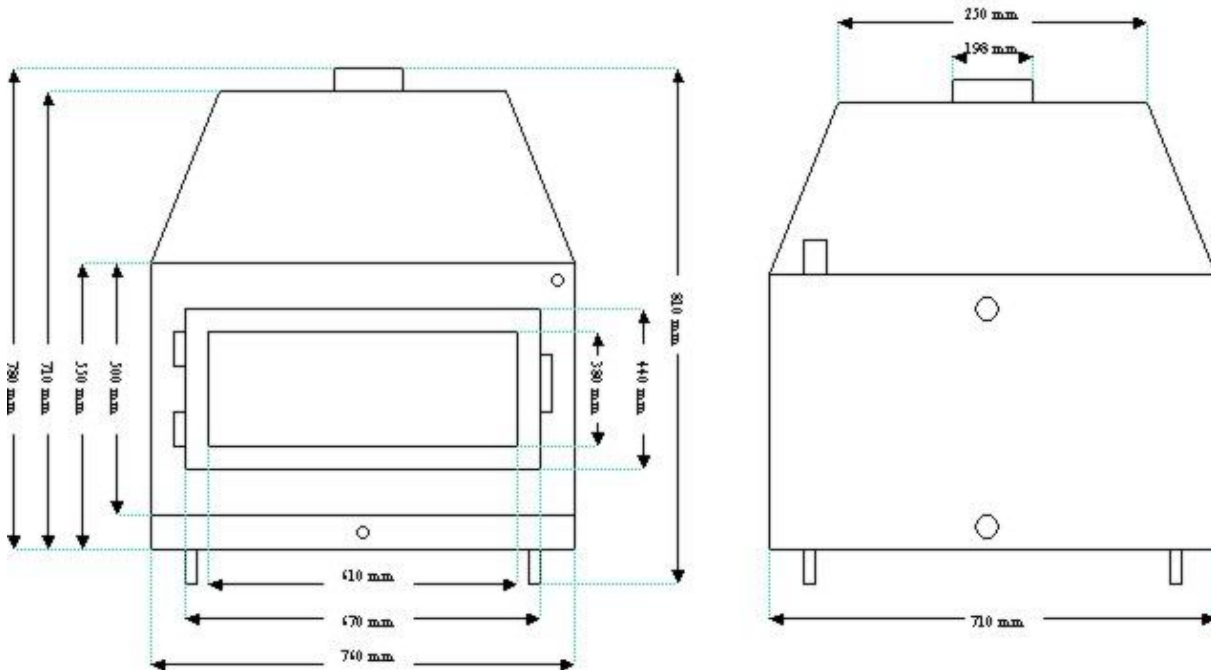
Wymiary poglądowe kominka 24 kW
